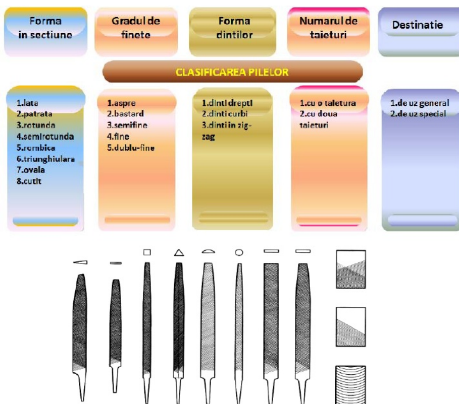
Fig.7.2.1.Pile(după forma în secțiune)
