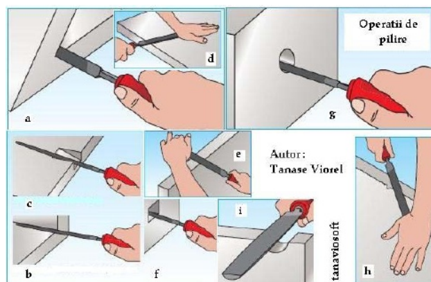
Fig.7.4.Metode de pilire
