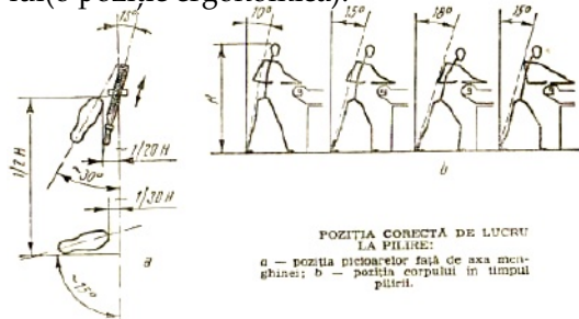
Fig.7.4.3.Poziția ergonomică
