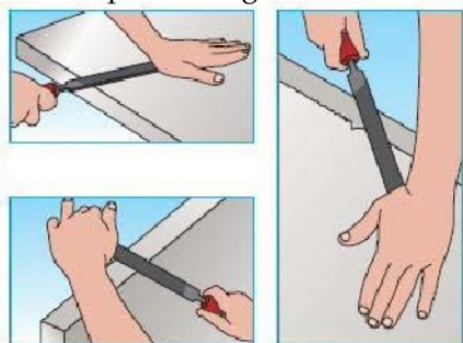
Fig.7.4.1.1.Pilirea de degroșare
