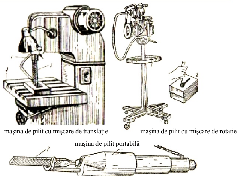
Fig.7.3.1.Mașini de pilit
