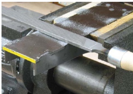
Fig.7.4.2.Fixarea piesei
