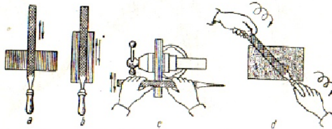
Fig.7.4.1.6. Pilirea de finisare
