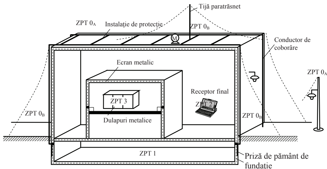
Fig. 4.6 – Zonele de protecție la supratensiuni de trăsnet.
