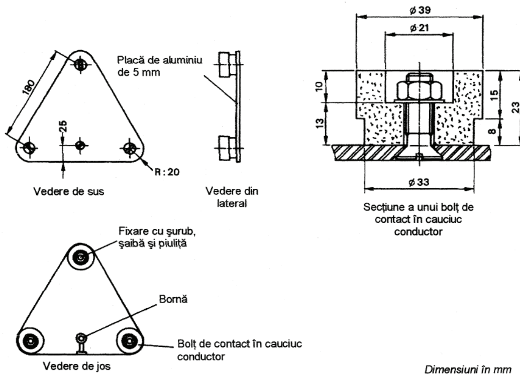
Fig. 8.1.1. – Electrode de încercare 1
