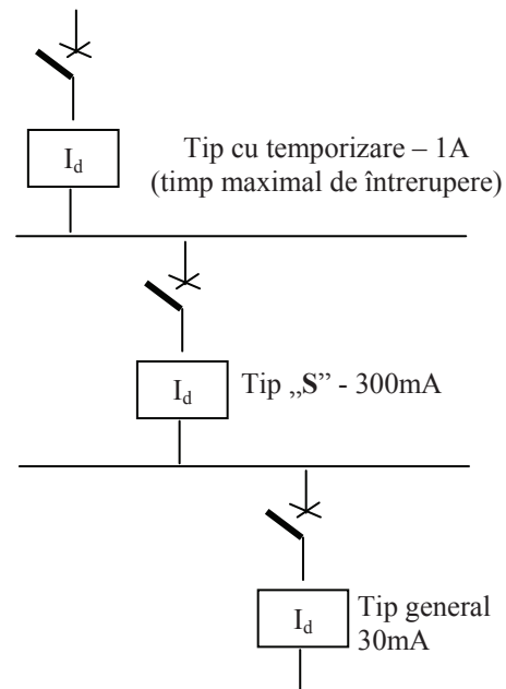
Fig. 4.2. Exemplu de circuite cu trei niveluri de selectivitate
