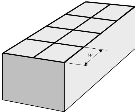
a – Dispozitiv de captare al unei IPT pe o structură cu acoperiș terasă
